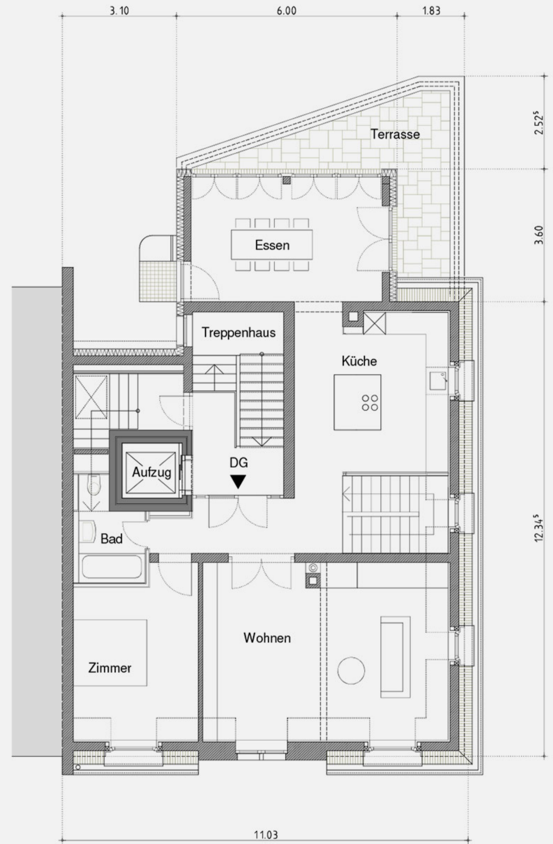
Dachgeschoss
